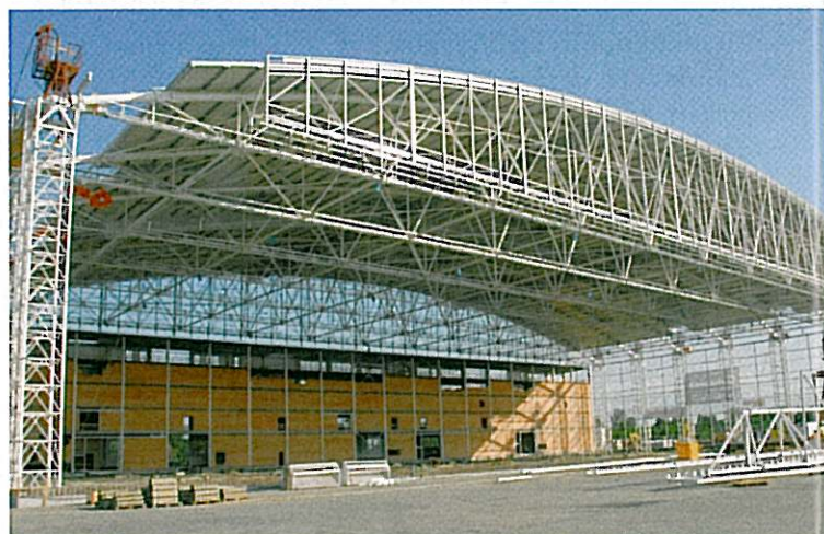
▲ Nosná ocelová konstrukce hangáru v Ostravě – Mošnově
