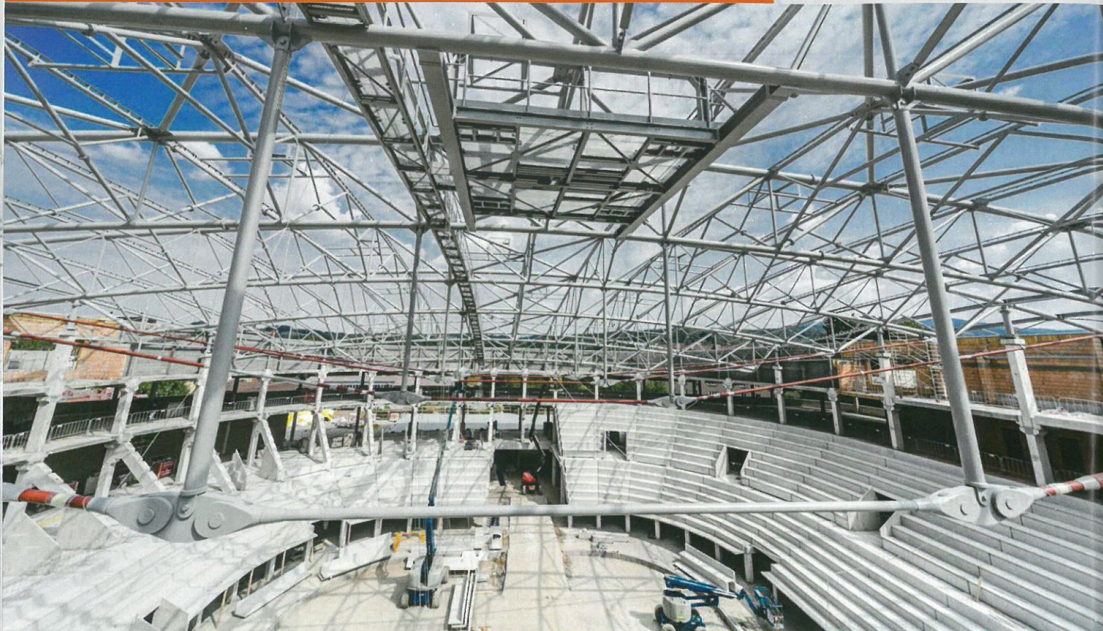
▲ Werk Arena Třinec – ocelová konstrukce zastřešení
