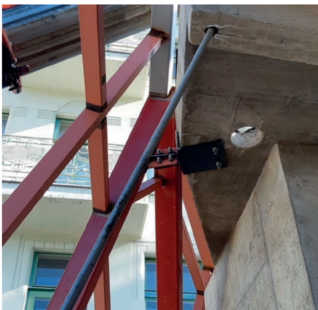
Detail kotvení
