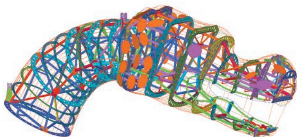
Obr. 3 – Detail konstrukce hlavy s přípojnými místy pro instalaci vnějších doplňků
