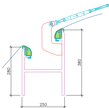
Tvar příčného řezu obvodových prvků a osazení lišt ETFE
